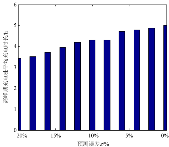
图 6 充电桩高峰期平均充电时长
