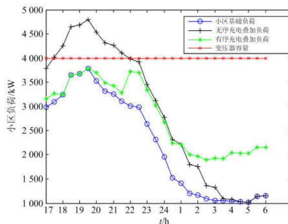
图 5 第一阶段负荷优化曲线
