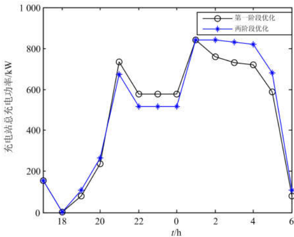
图 8 预测误差 \varepsilon 为 10%
