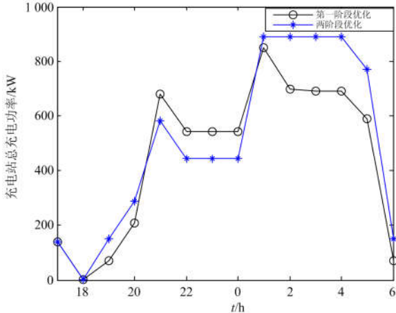
图 7 预测误差 \varepsilon 为 20%
