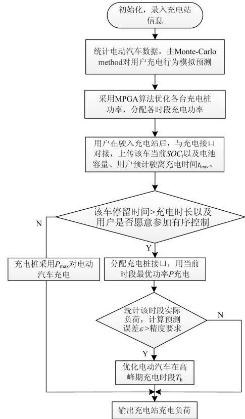
图 2 两阶段有序充电策略算法
