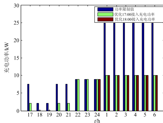
图 4 各时段充电功率大小
