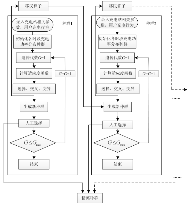
图3 MPGA 算法流程图
