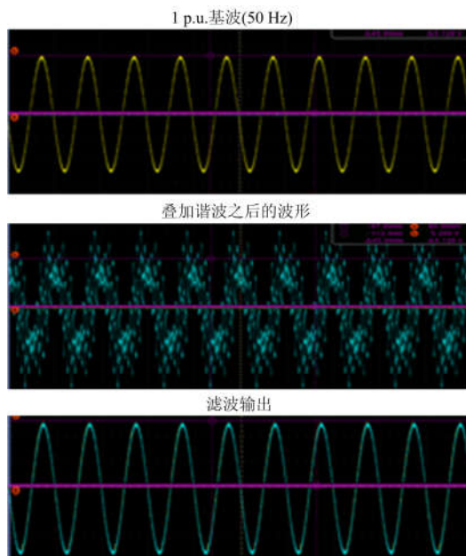
图 5 滤波器功能验证结果
