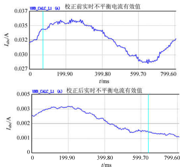
图 6 工程应用中滤波器使用效果
