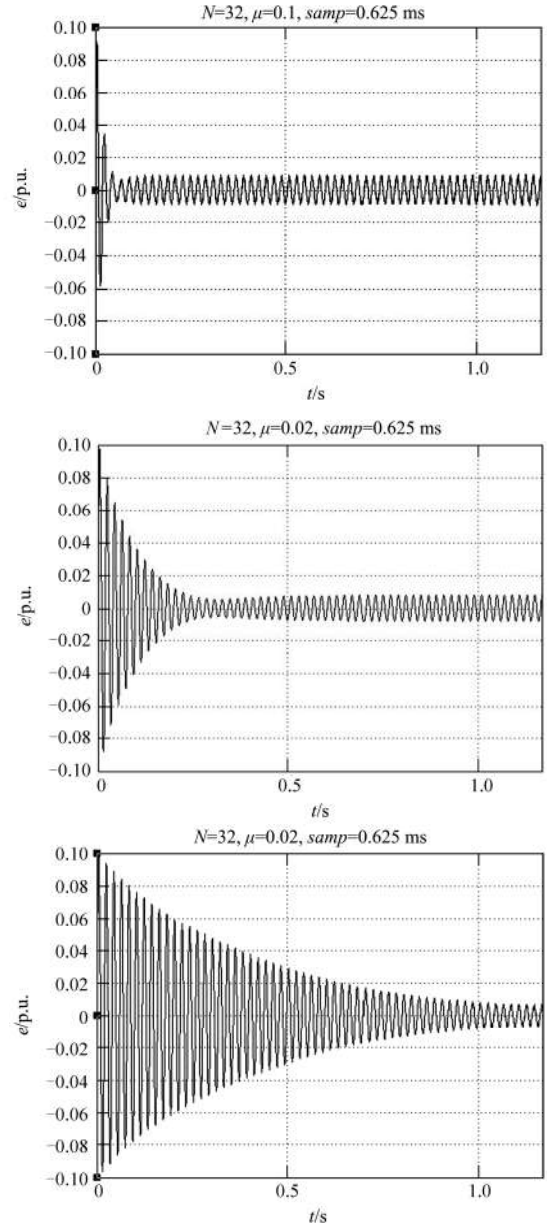
图 4 不同迭代步长时滤波器仿真输出
