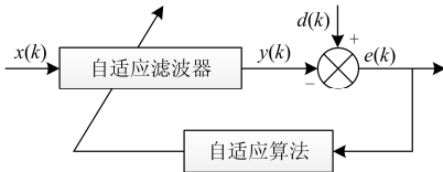
图 2 自适应滤波器基本结构图
