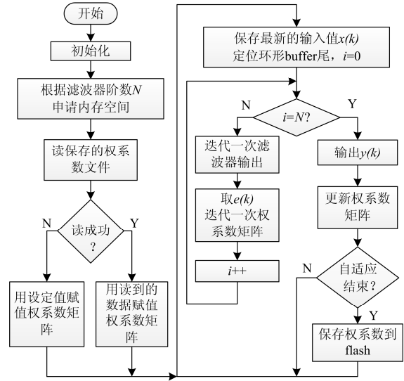
图 3 HCM3000 中 LMS 自适应滤波器算法流程图
