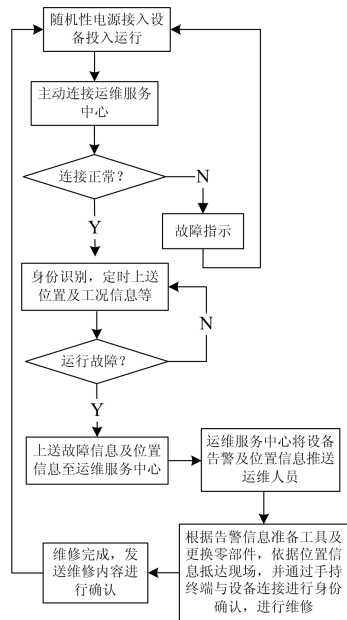
图 9 故障维修流程图
