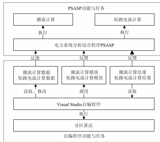
图 3 Visual Studio 与 PSASP 功能、任务示意图
