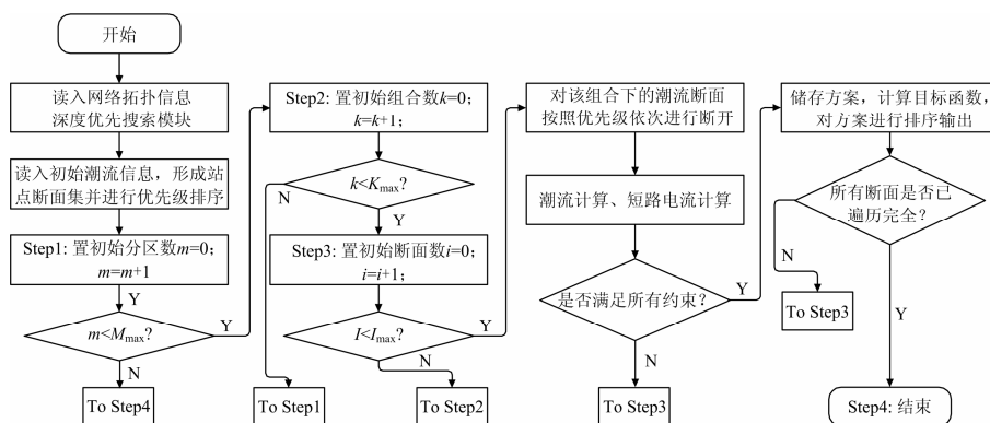
图 4 分区计算流程图
