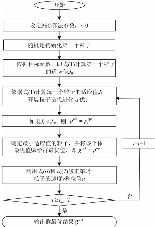
图 1 本文算法流程图
