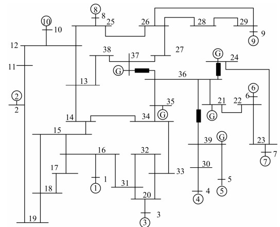
(b) 3台SRFCL的安装方案示意图
