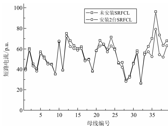
图4 2台SRFCL安装前后的全网母线短路电流对比
