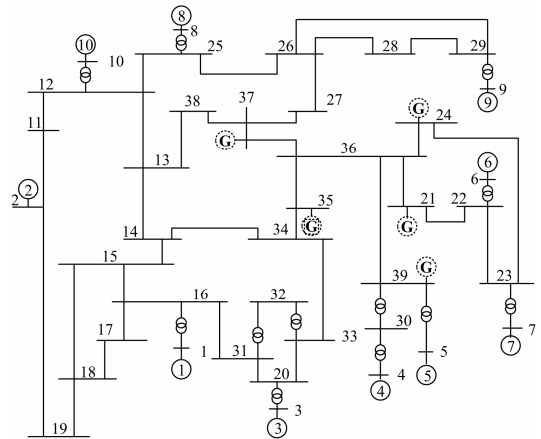
图 2 一个修改的IEEE39节点测试系统
