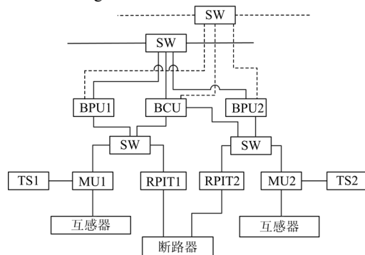
图 4 基于 PRP 的过程层总线
