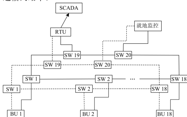
图 3 基于 PRP 的站控层总线
